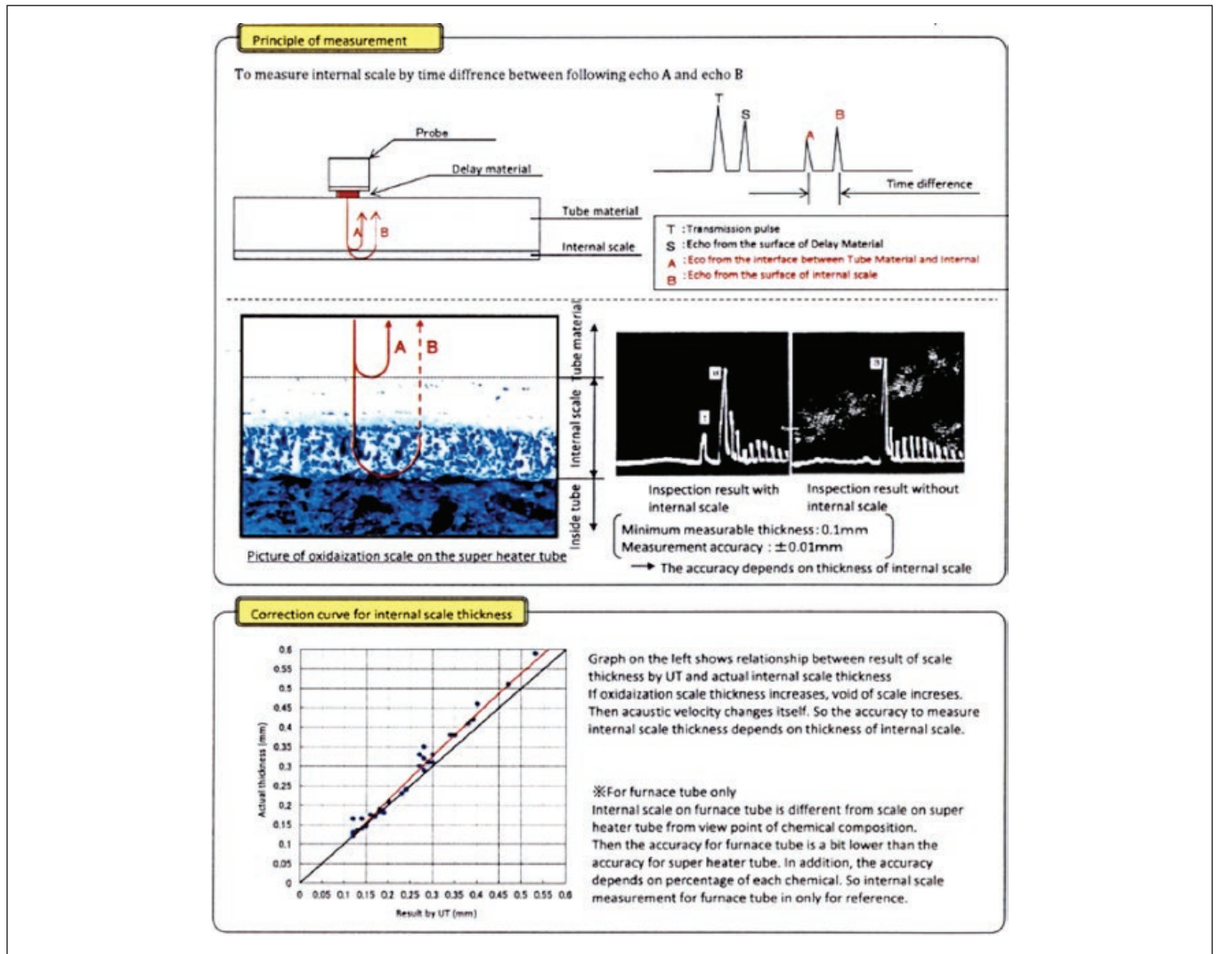
Figura 3. Princípio da medição da espessura da camada de óxidos via ultrassom Fonte: Mitsubishi Hitachi Power Systems Co, Ltd, Japão [6]
