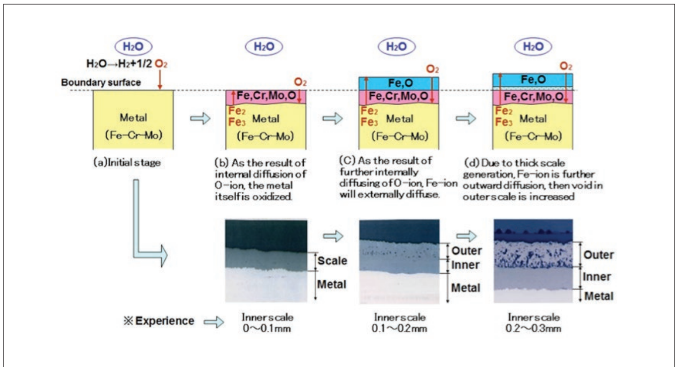
Figura 2. Mecanismo de formação da camada de óxidos no interior de tubos de aço liga em caldeiras Fonte: Mitsubishi Hitachi Power Systems Co., Ltd, Japão [6].
